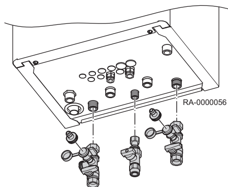
Rys.14 Instalacja zaworów separujących
