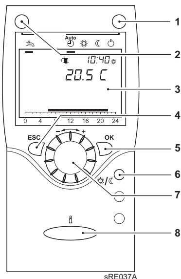
Rys.5 Interfejs obsługi regulatora pokojowego RGT
