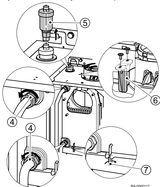
Rys.40 Demontaż wymiennika ciepła
