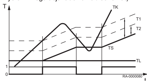
Rys.31 Regulacja ładowania / schemat)
