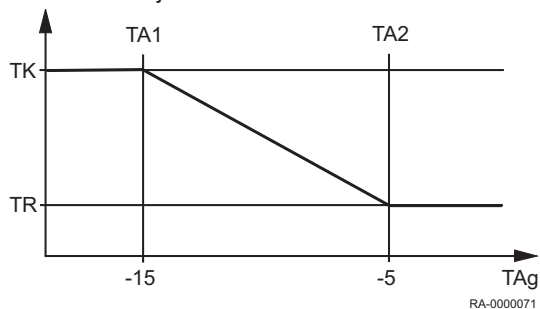
Rys.26 Zwiększanie obniżonej wartości zadanej
