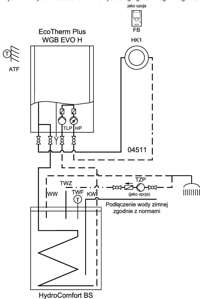
Rys.10 Przykład zastosowania: Pompa obiegu grzewczego z regulatorem pokojowym z regulacją temperatury w zasobniku
