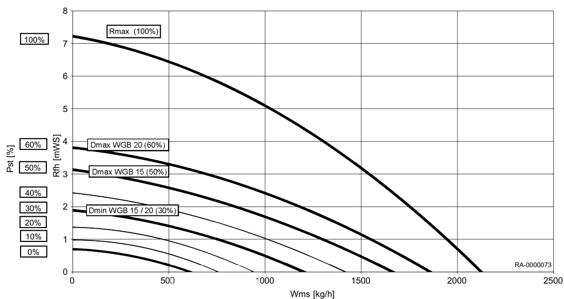
Rys.1 Łączne ciśnienie dynamiczne WGB EVO 15 — 20
