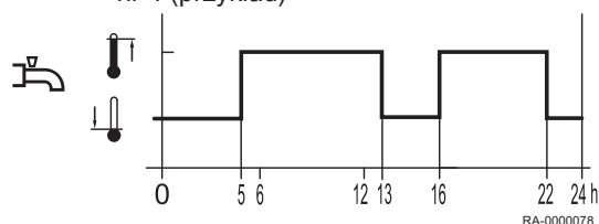
Rys.29 Odblokowywanie w zależności od programu czasowego przełączania nr 4 (przykład)
