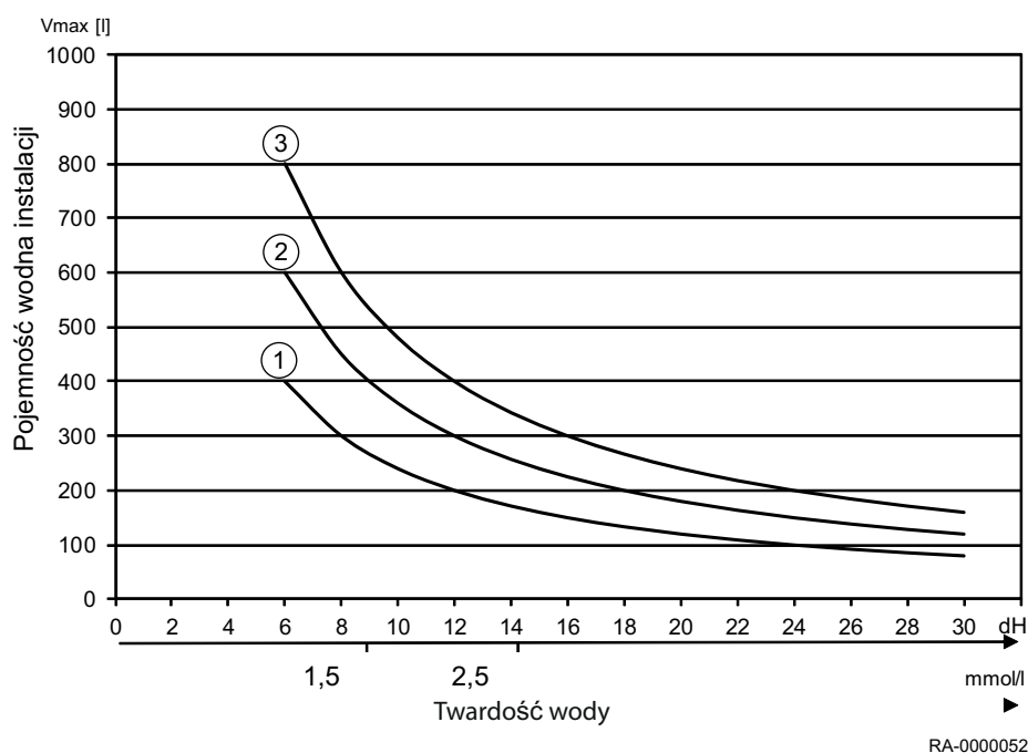
Rys.8 Wykres twardości wody
