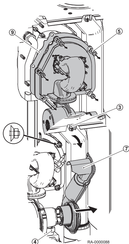
Rys.39 Demontaż palnika gazowego
