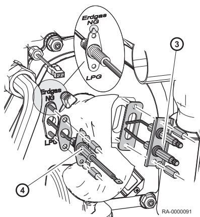
Rys.38 Demontaż elektrody zapłonowej i jonizacyjnej
