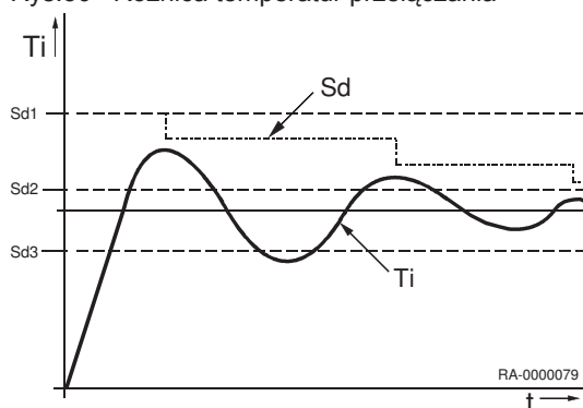
Rys.30 Różnica temperatur przełączania
