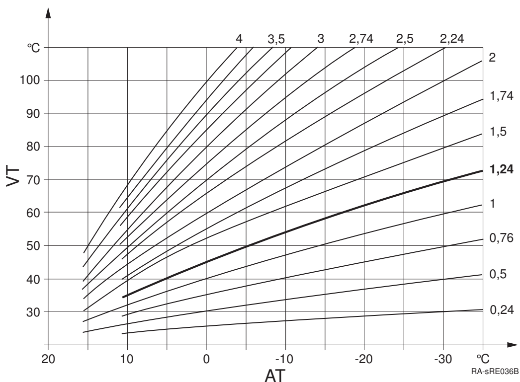
Rys.21 Wykres krzywej grzewczej
