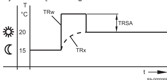
Rys.24 Zwiększone ogrzewanie
