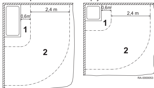
Rys.9 Odstępy izolacyjne w łazienkach i pomieszczeniach z prysznicami
