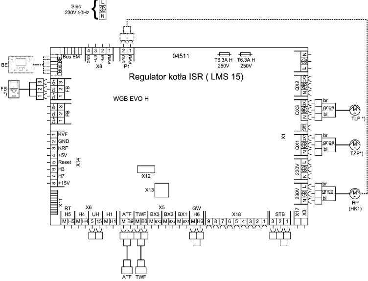
Rys.11 Schemat elektryczny
