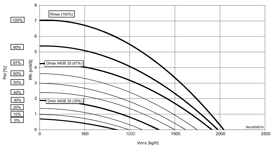
Rys.2 Łączne ciśnienie dynamiczne WGB EVO 28
