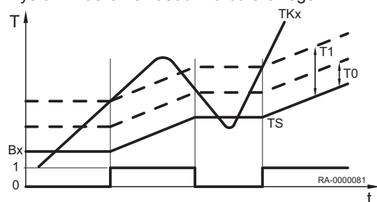
Rys.32 Zasilanie zasobnika buforowego
