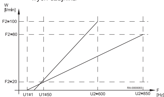
Rys.34 Przykład dla dwóch różnych krzywych czujnika
