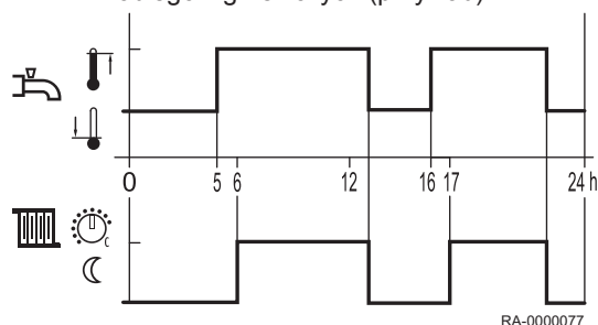
Rys.29 Odblokowywanie w zależności od programu czasowego przełączania nr 4 (przykład)
