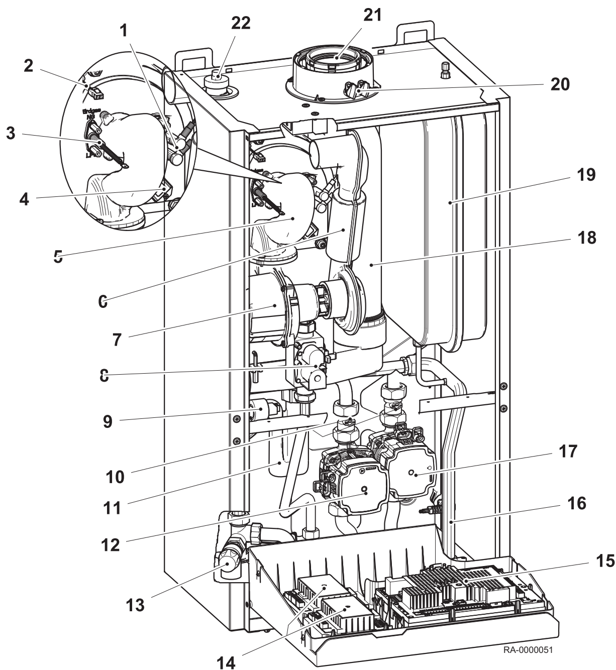
Rys.4 Widok kotła WGB EVO (bez przedniej ścianki i pokrywy regulatora)
