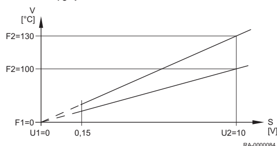
Rys.35 Przykład zapotrzebowania na ciepło 10 V
