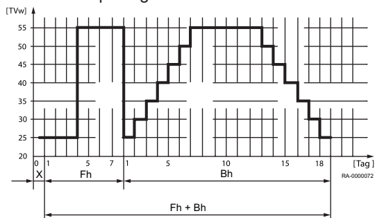
Rys.27 Profil temperaturowy funkcji osuszania podłogi
