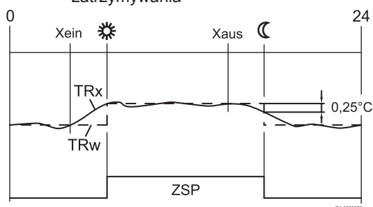
Rys.25 Kontrola optymalnego uruchamiania i zatrzymywania
